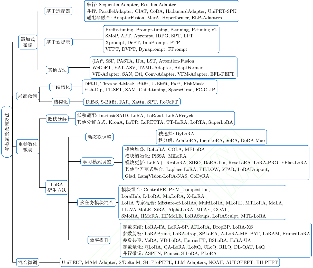
图3 PEFT方法分类图
