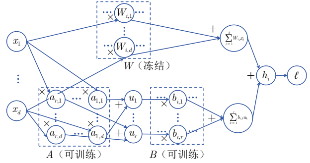
图 4 LoRA 模块的计算示意图
