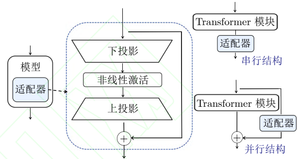
图 2 适配器结构图示
